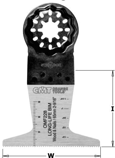
OMF228 STARLOCK
