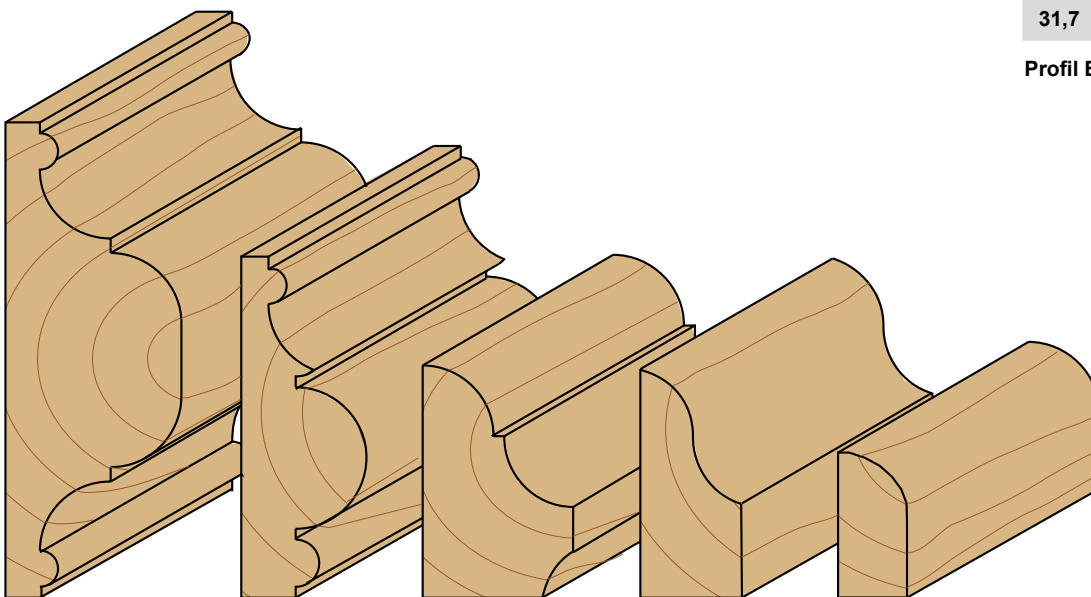
4 Arbeitsgänge
