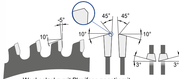
Wechselzahn mit Plexifase negativ mit wechselseitigem Achswinkel (W/Fa neg., AW), HW
