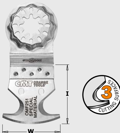
OMF251 STARLOCK
