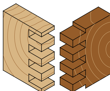
Fingerzinken
