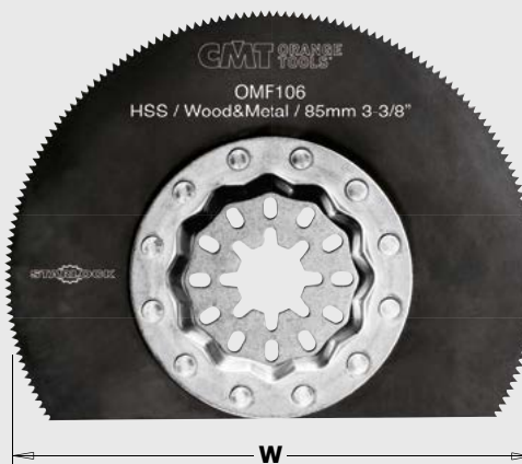
OMF106 STARLOCK
