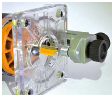
Kantenführung mit Delrin®-Anlaufing zur Verhinderung von Kratzspuren am Werkstück
