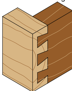
Halbverdeckte Zinkenverbindung
