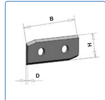
Wendepplatte mit Fase, 2 Schneidkanten
