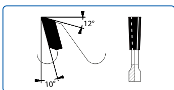
Abb.: Flachzahn (F),zweiteilig
