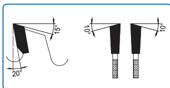
Abb.: Wechselzahn mit Fase (WS)
